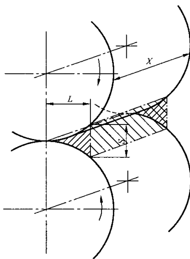
图 2 压延辊筒的吸入区
