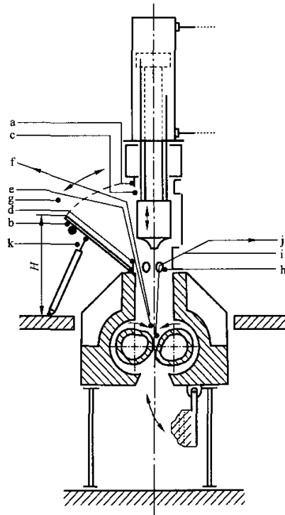
图 2 在加料区和其他加料开口处机械危险的位置
