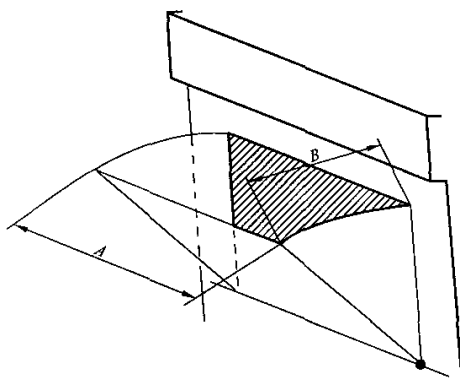
图 8 加料前门开口尺寸
