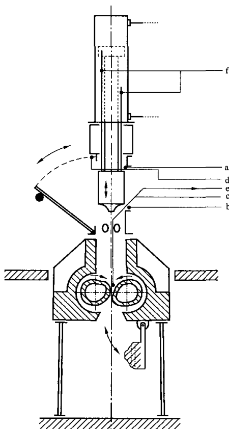
图 3 加料斗后开口处机械危险的位置
