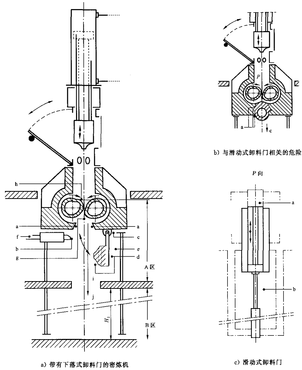
图 4 卸料区危险位置
