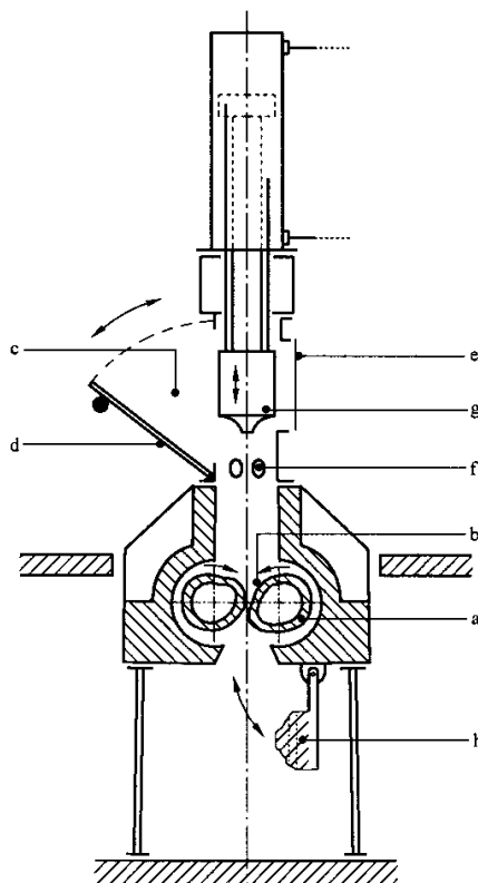
图 1 密炼机主要部件图
