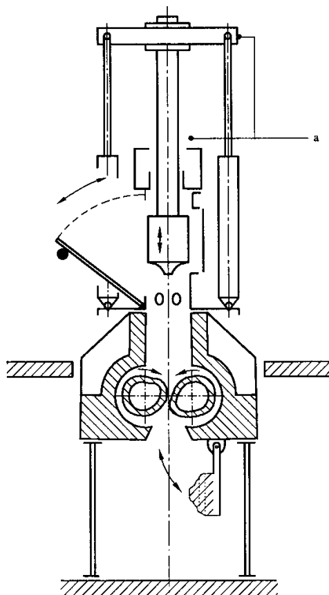
图 6 压砷运动引起危险的位置
