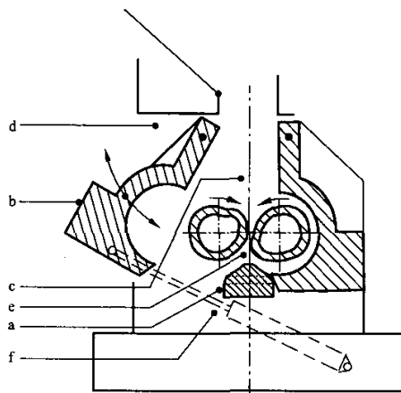
图5 卸料区的机械危险位置(通过密炼室的开口部分卸料)
